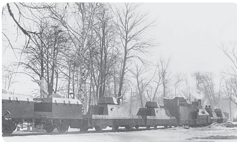
Второй бронепоезд типа БП-43 «Советский железнодорожник», изготовленный Коломенским заводом в феврале 1943-го года. На первом плане стоит платформа ПВО-4. За ней две бронеплощадки с башнями танка Т-34-76. В центре бронепаровоз, который включался в работу только в боевом выходе.
